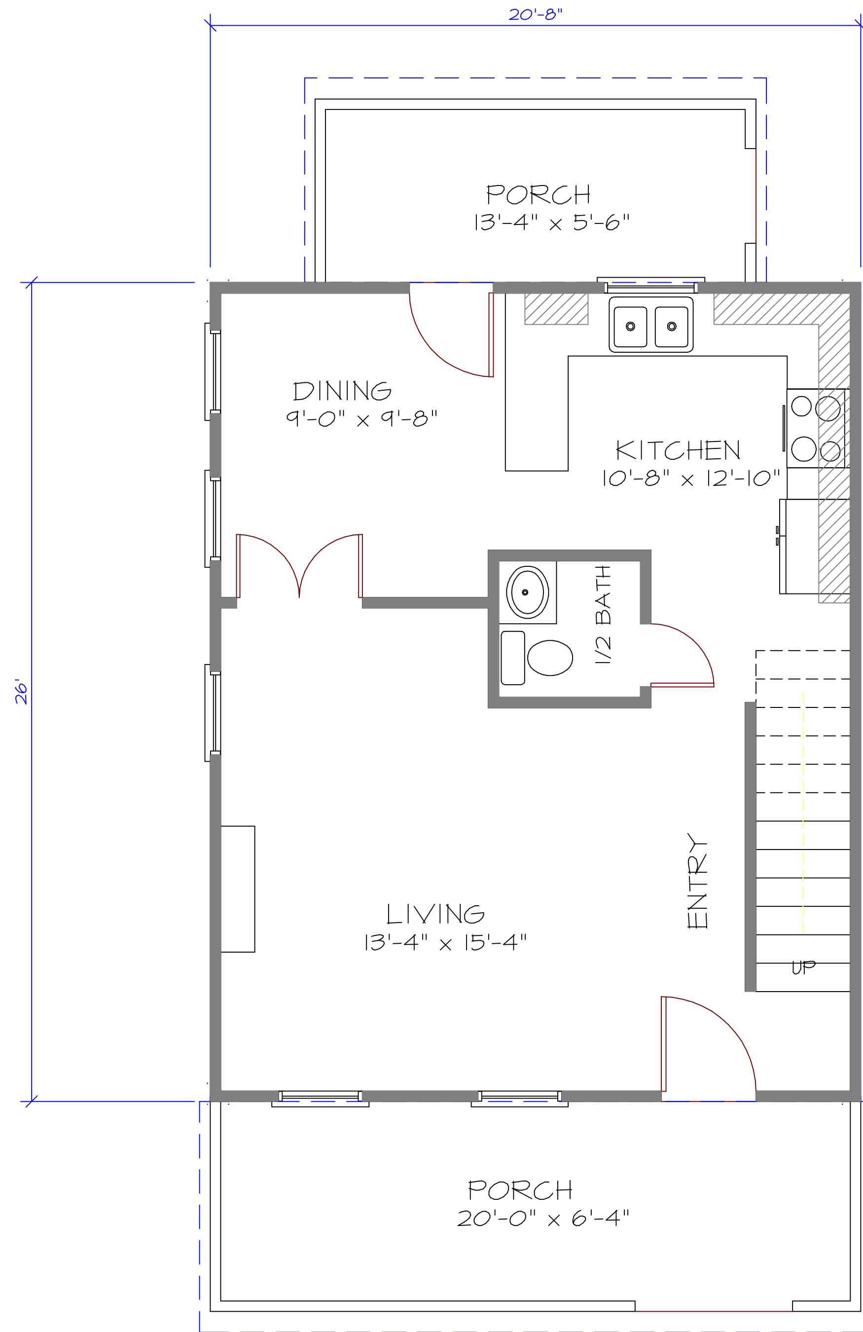
FIRST FLOOR PLAN N.T.S.
